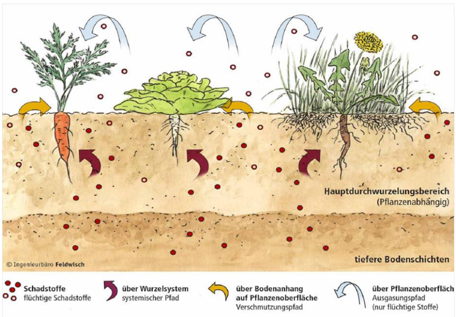
Abbildung 1: Schadstoffübergang Boden Pflanze (Quelle: Ingenieurbüro Feldwisch)
